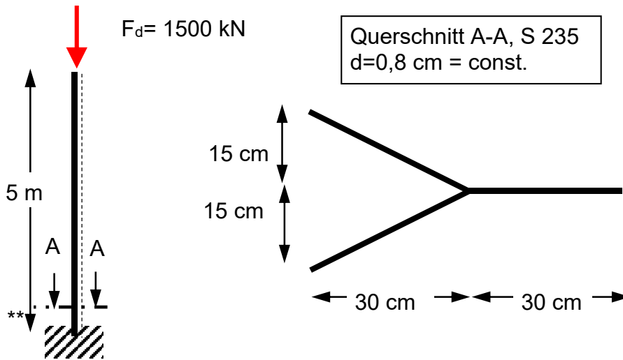
Bild 5-11: Beispiel 3 zum Biegeknicken
