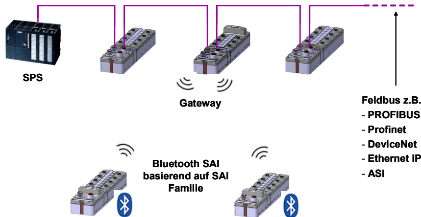
Abb. 3: Feldbus-System mit zusätzlichen Bluetooth-Funk-SAI's
