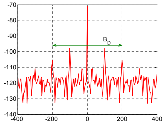
Abb. 16: Doppler-Spektrum in dB für die Umgebung IND 4 von -400 Hz ... 400 Hz
