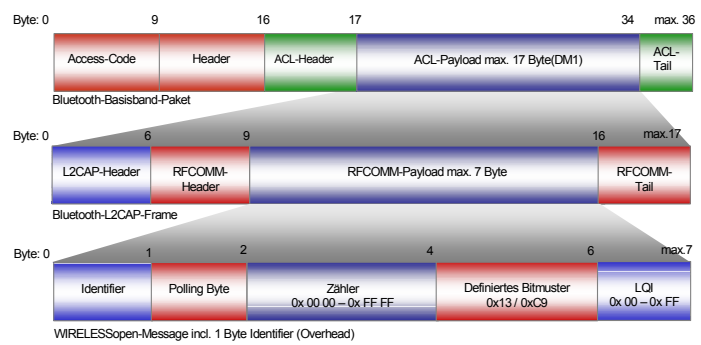
Abb. 5: Protokollaufbau der WIRELESSopen-Message (als Antwort des Slaves)
