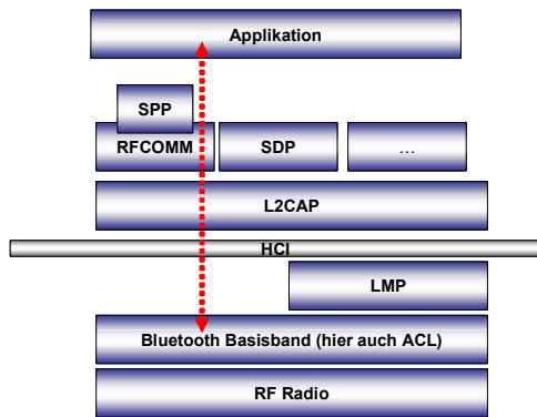
Abb. 4: Kommunikationspfad durch den Bluetooth Protokoll Stack
