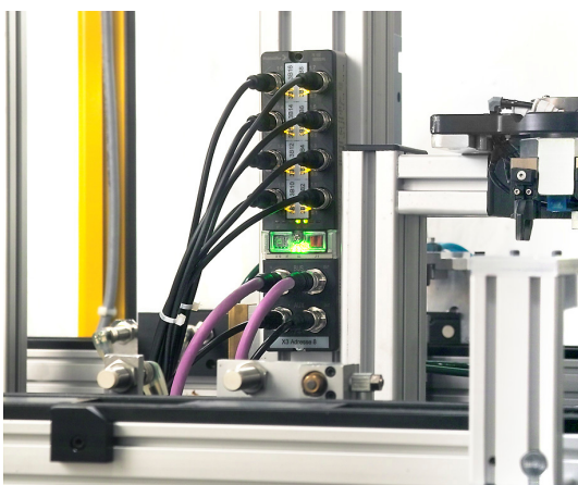
Abb. 1: Kabelgebundenes Sensor-Aktor-Interface (SAI) in einer Automatisierungsapplikation
