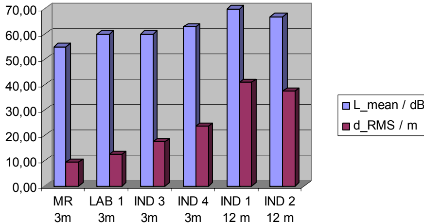
Abb. 14: Mittlere Dämpfung und Delay Spread
