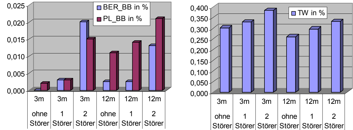
Abb. 11: Kabelgebundene Messwerte ohne / mit WLAN Störer
