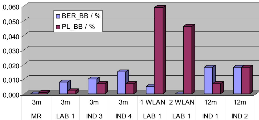
Abb. 13: Paketverluste und Bitfehlerrate im Basisband
