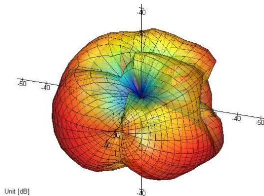
Abb. 6: Richtdiagramm SAI-Stabantenne für horizontale Polarisation (0 ... -40 dB)
