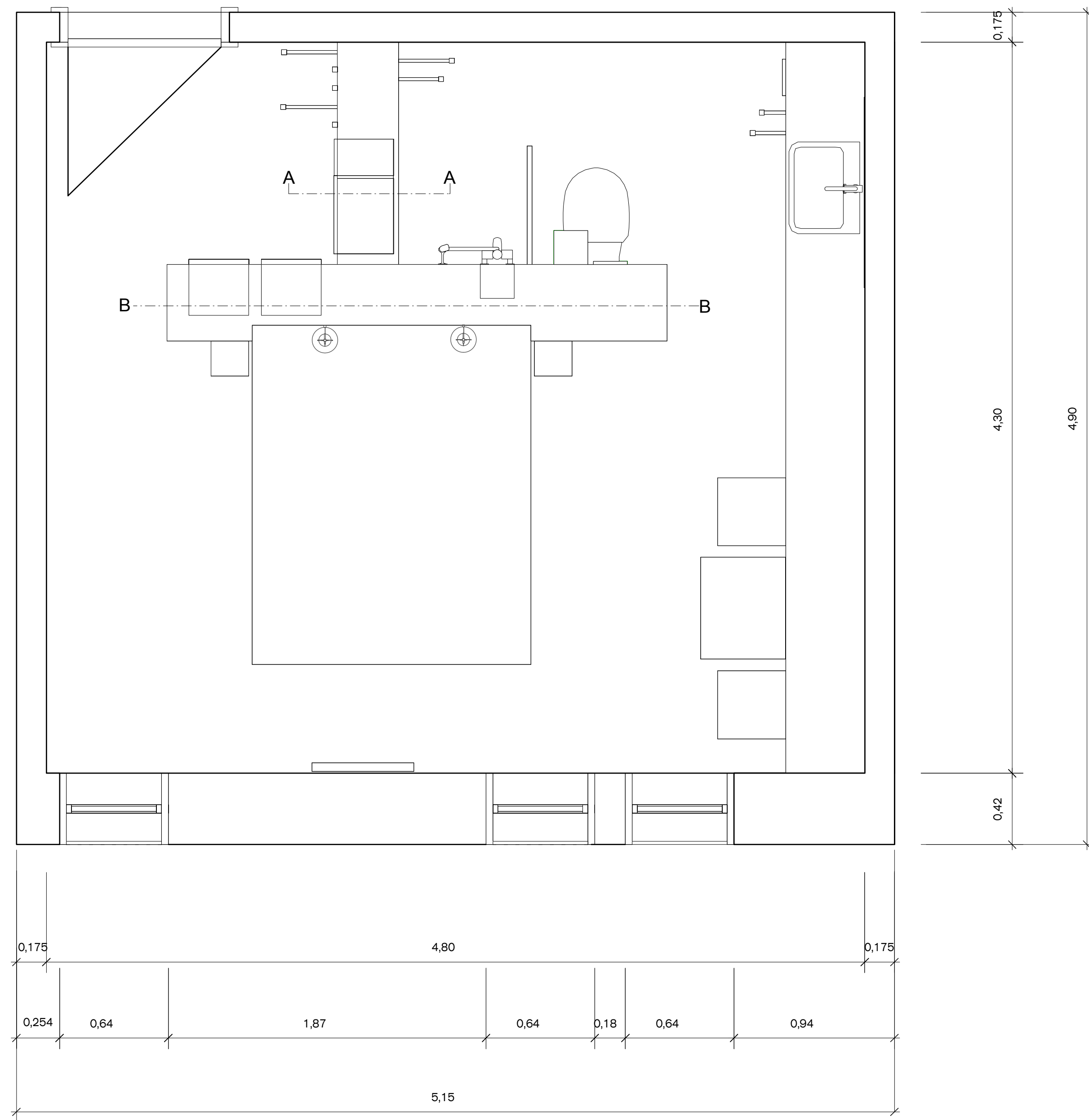
Grundriss OG 1:100 _ Zimmer 1:20
