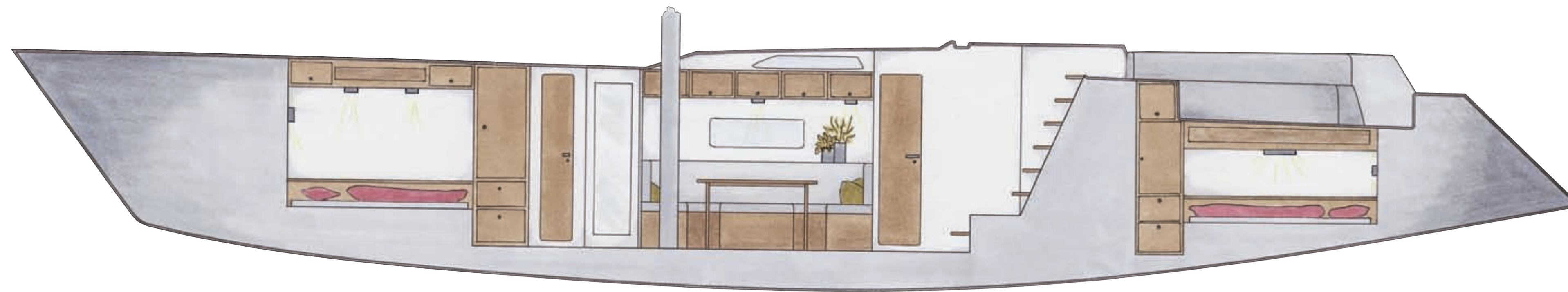
Schnitt A-A M 1:33 1/3
