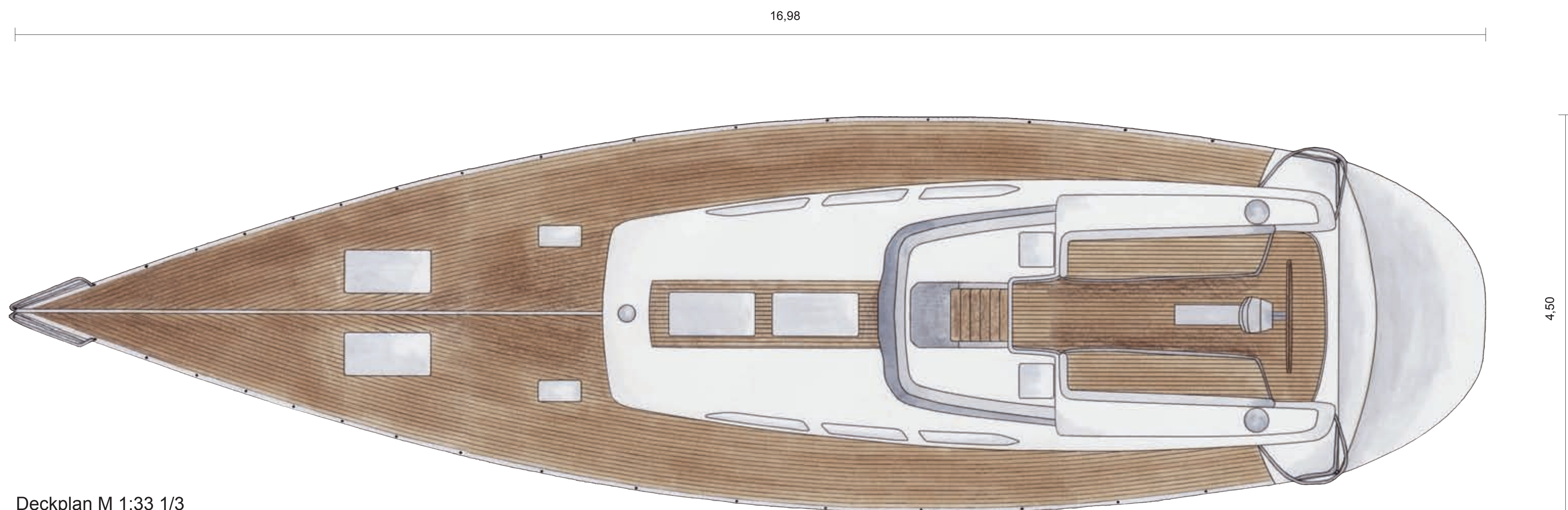
Deckplan M 1:33 1/3
