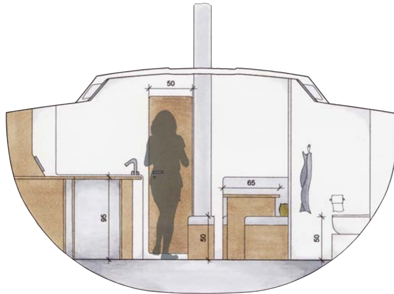
Spantenschnitt 3 M 1:25
