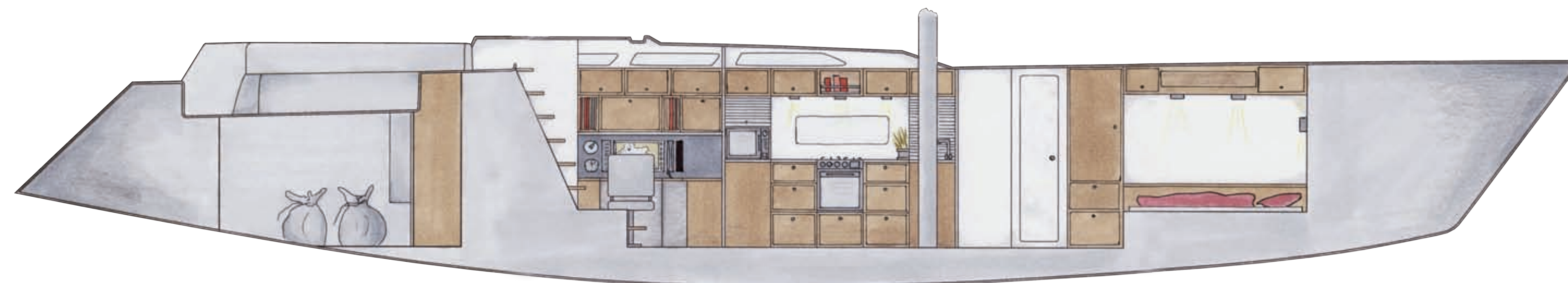
Schnitt B-B M 1:33 1/3
