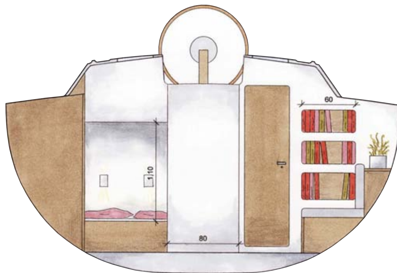
Spantenschnitt 4 M 1:25
