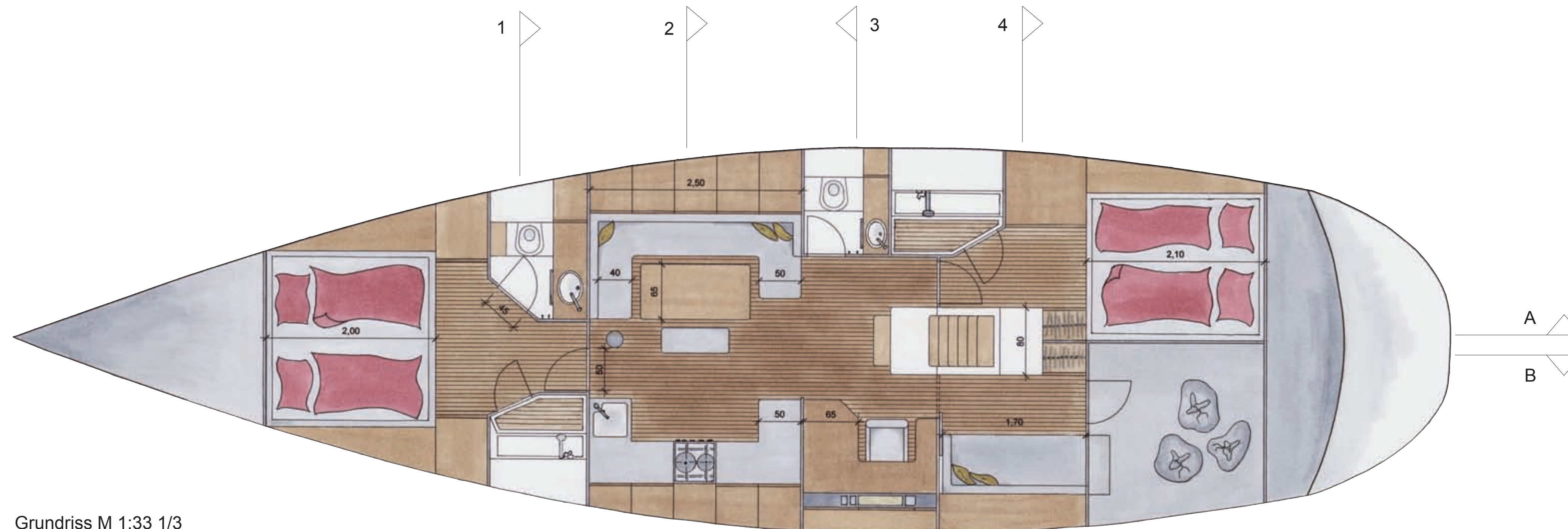
Grundriss M 1:33 1/3
