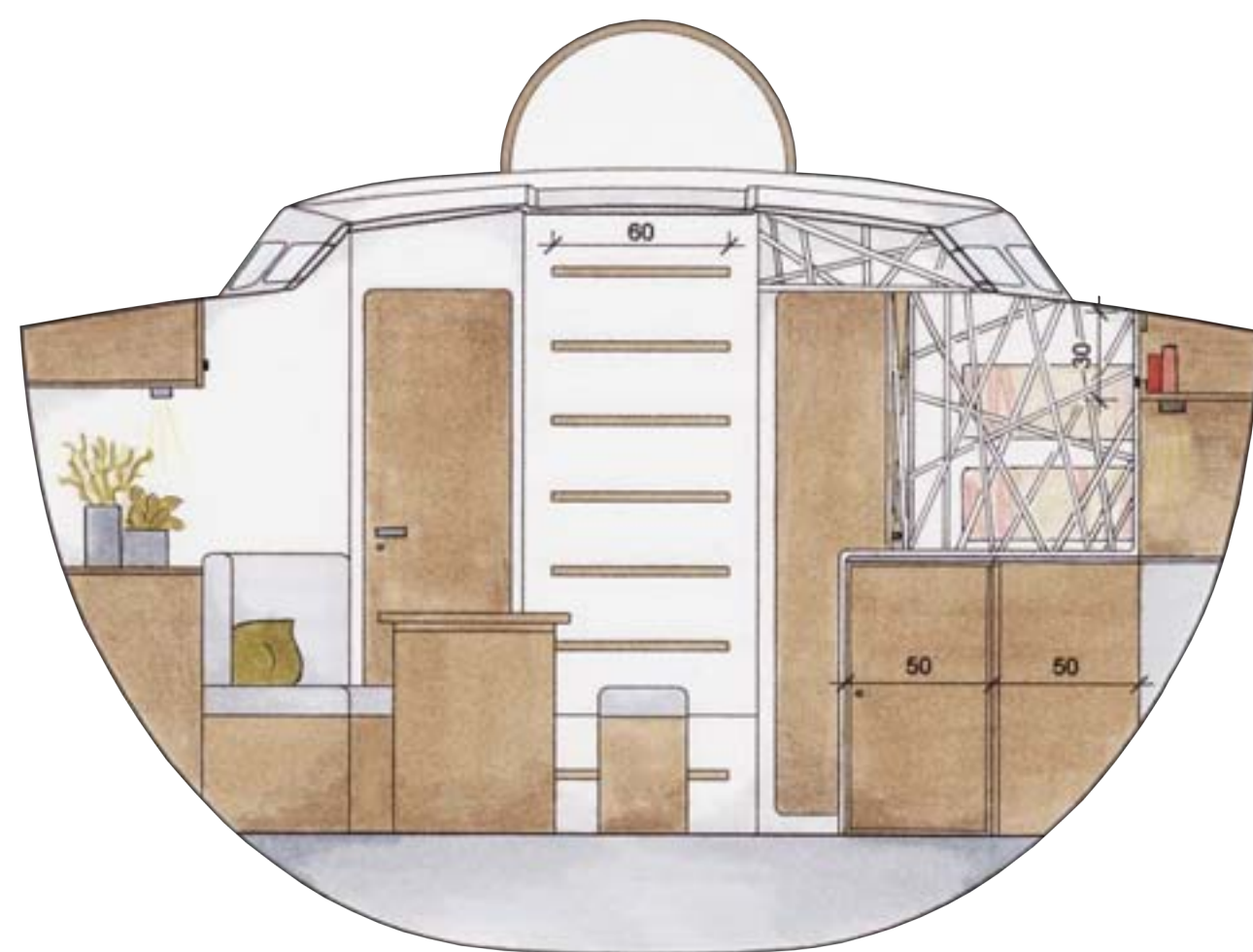
Spantenschnitt 2 M 1:25
