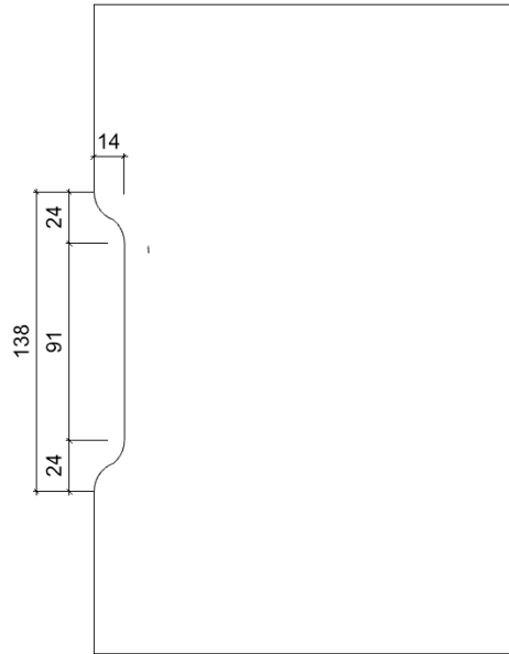
Vorderansicht
