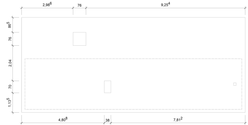
Draufsicht
