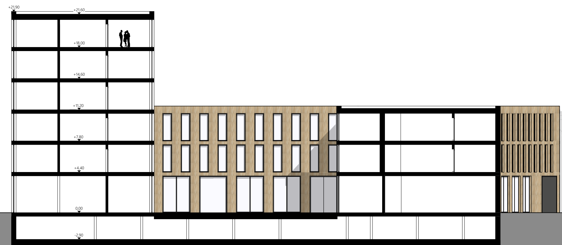
Schnitt D-D M. 1:250
