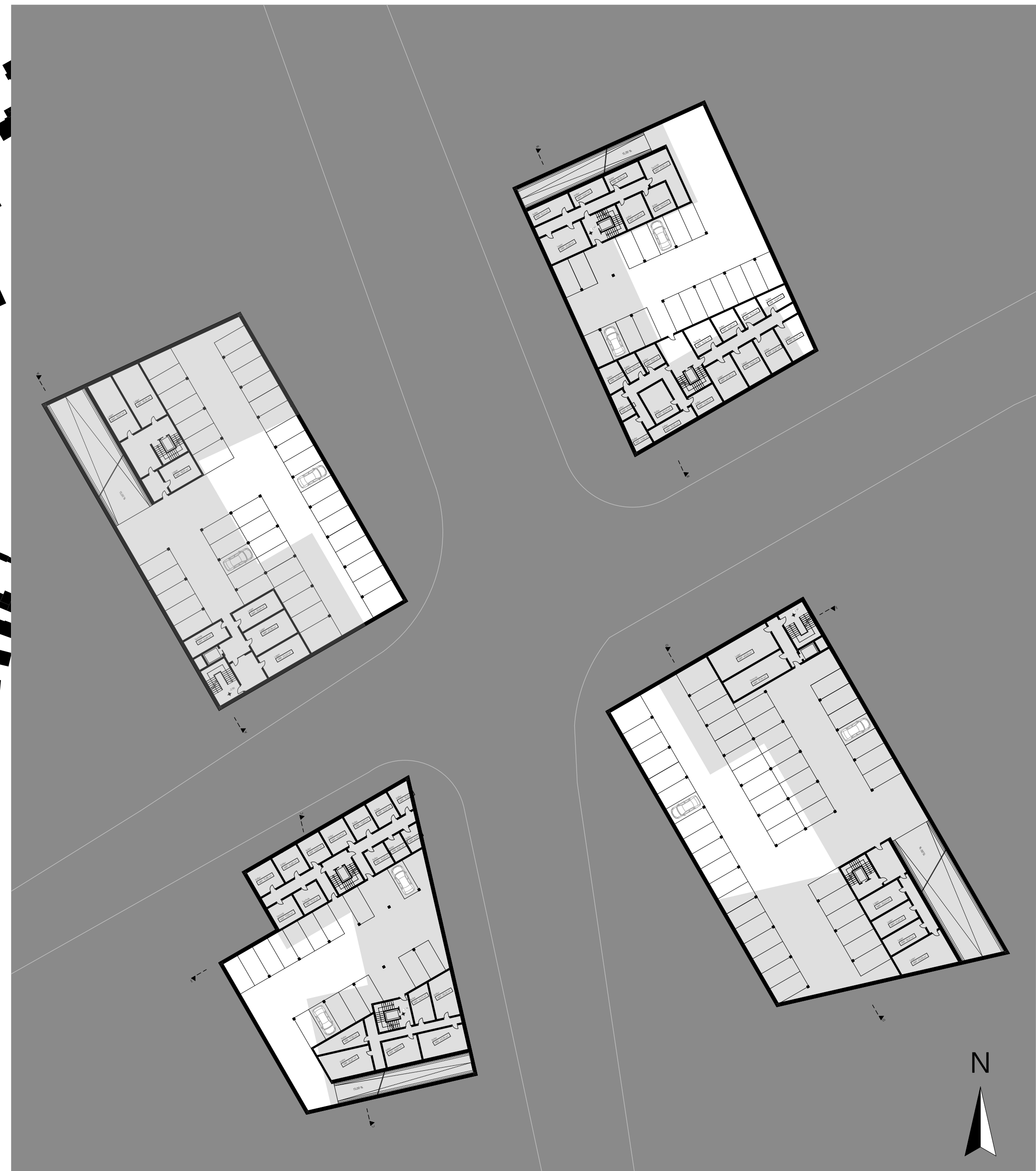
Tiefgarage M. 1:500
