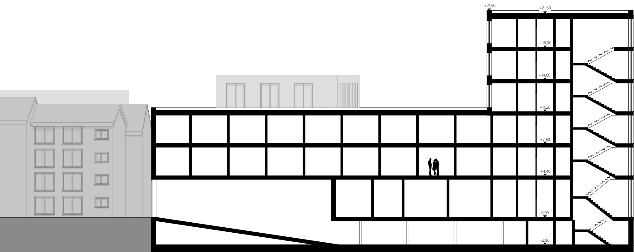
Schnitt A-A M. 1:250
