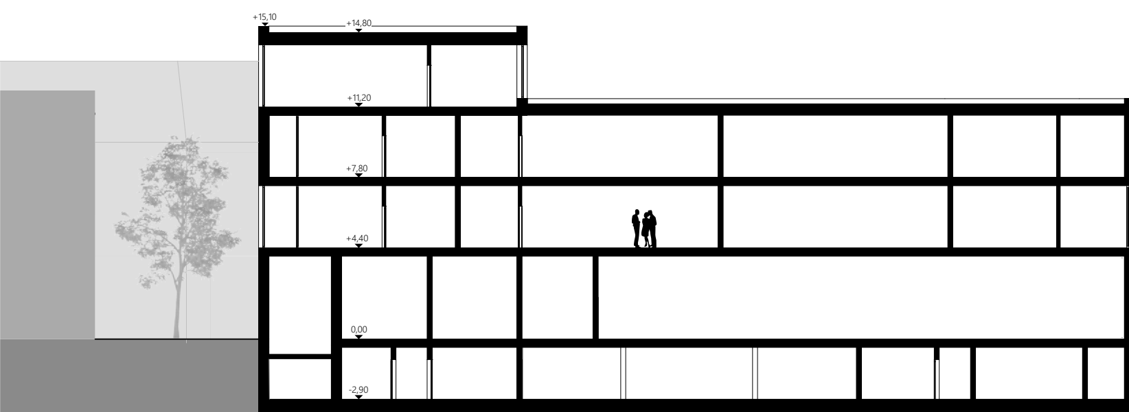
Schnitt B-B M. 1:250
