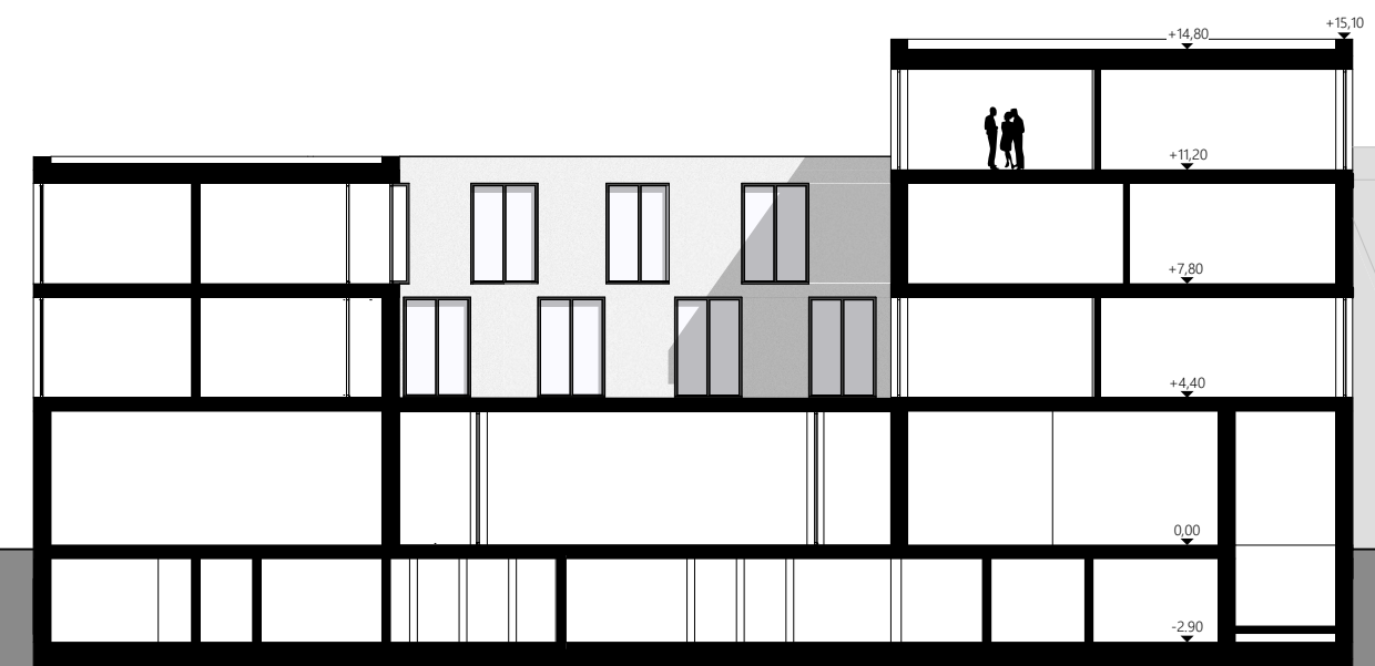
Schnitt C-C M. 1:250
