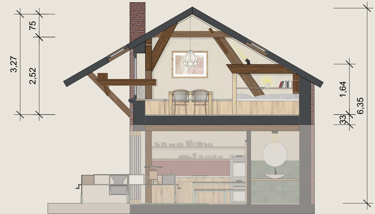
Schnitt D-D
