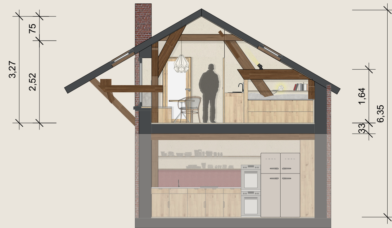
Schnitt C-C
