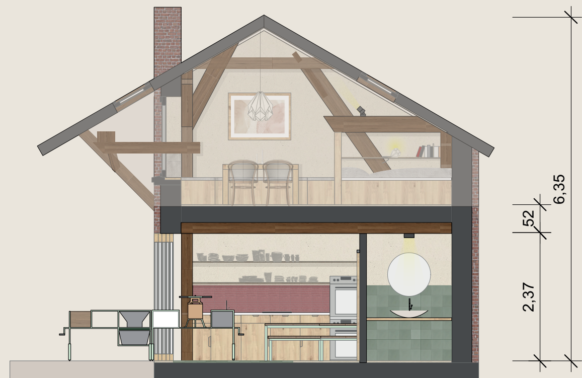
Schnitt D-D
