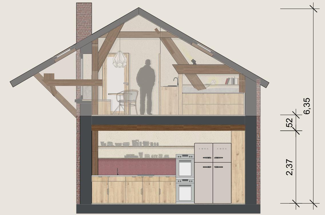
Schnitt C-C
