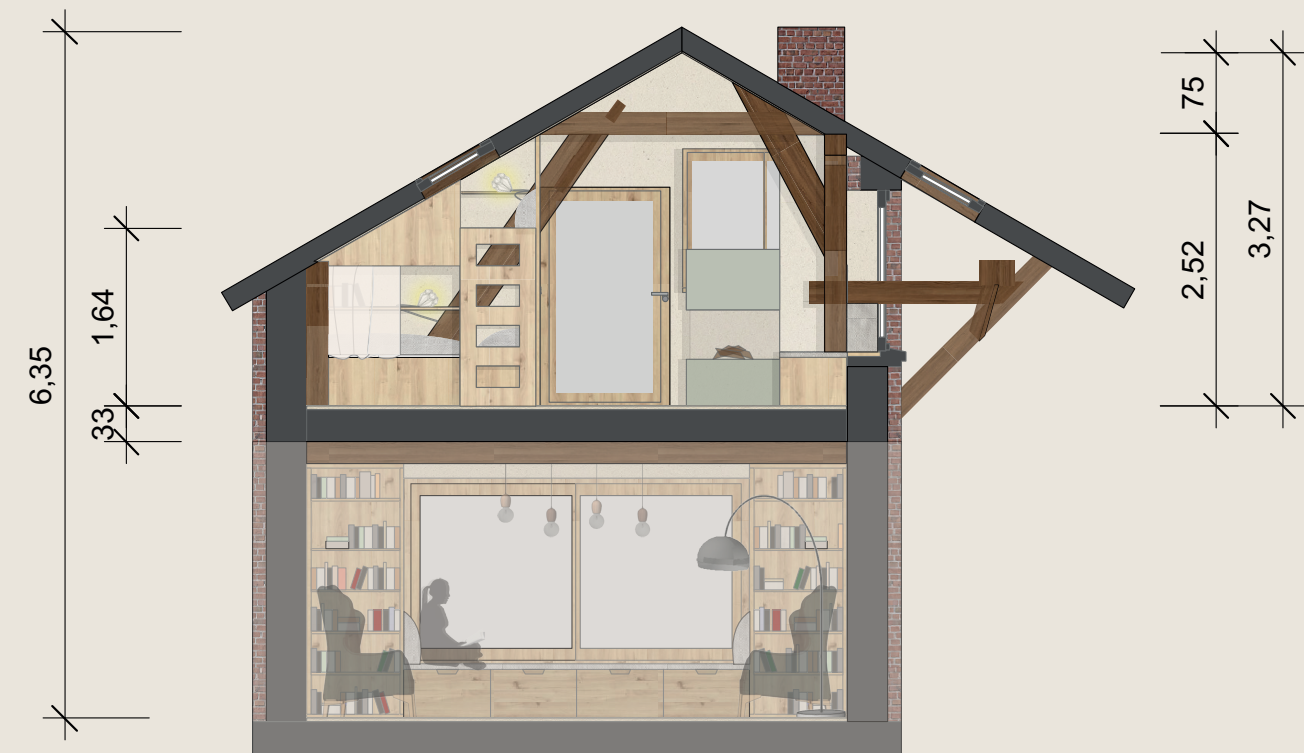
Schnitt E-E
