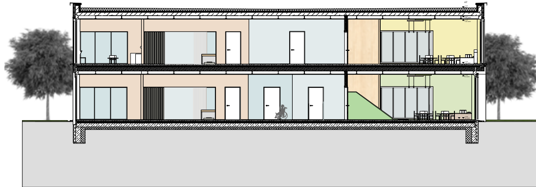
Schnitt A-A M 1:100
