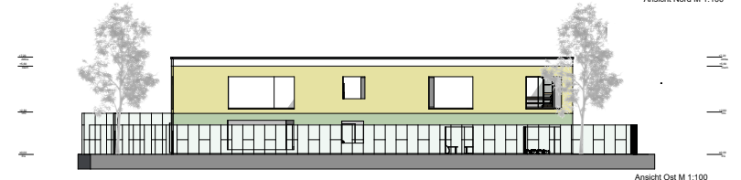
Ansicht Ost M 1:100
