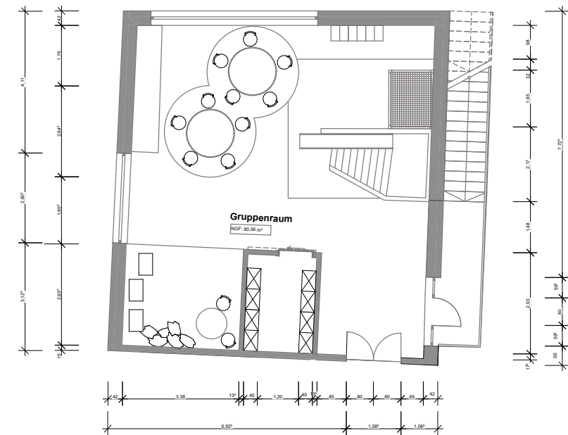
Grundriss Gruppenraum OG M: 1:100
