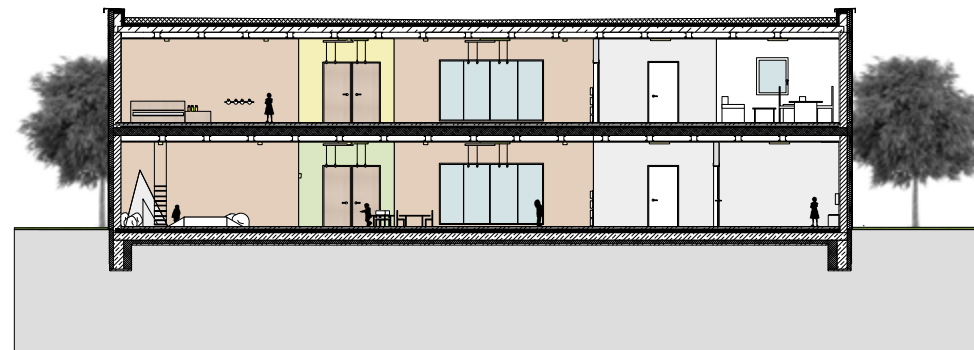
Schnitt B-B M 1:100
