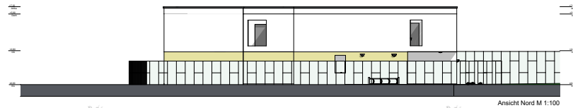
Ansicht Nord M 1:100
