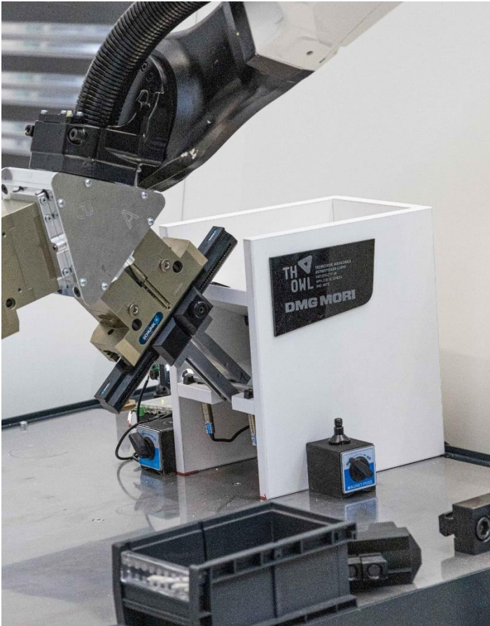
Automatisierte Vereinzelung von additiv gefertigten Rundzugproben
